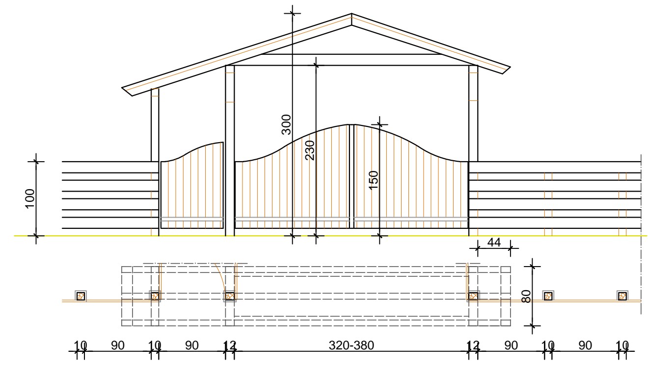
главна улазна капија R1:50
