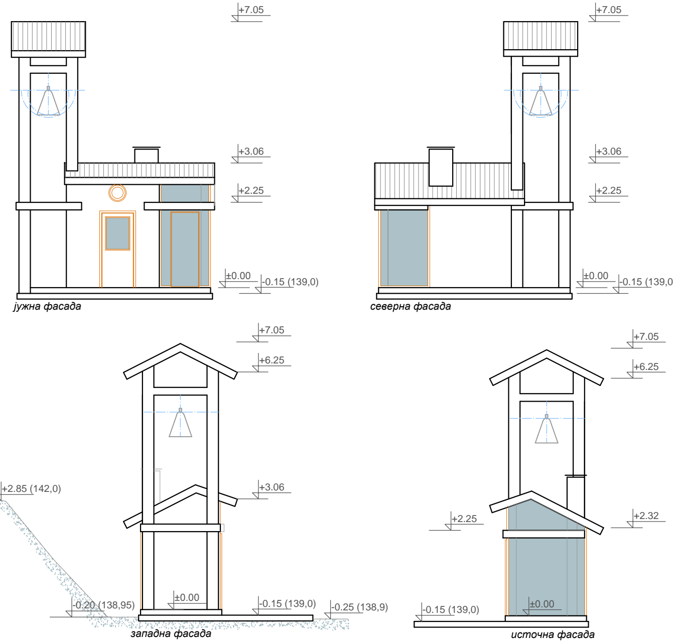
Јужна фасада, северна фасада, западна фасада, источна фасада
