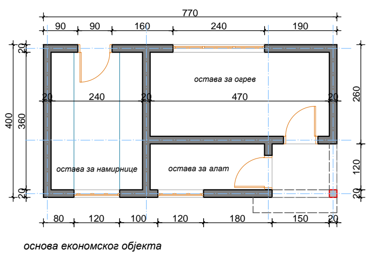
основа економског објекта
