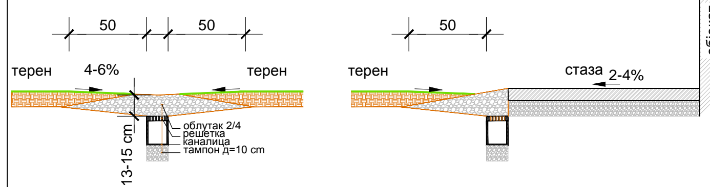
ДЕТАЉ КИШНЕ КАНАЛИЗАЦИЈЕ R1:25
