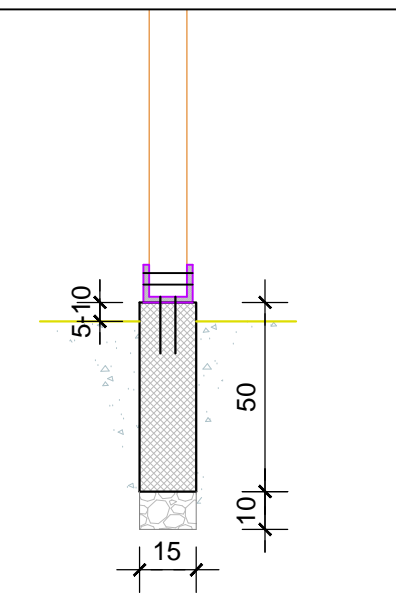
деталј темеља стуба оградe R 1:20
