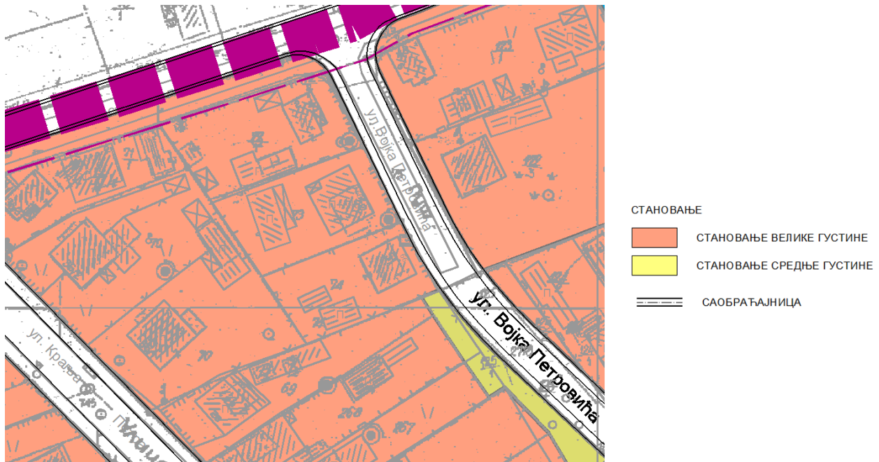
Графички прилог 2. Извод из Плана детаљне регулације „Зона I Централна“ Лајковац („Службени гласник општине Лајковац“ број 4/2010) - примењује се графички део плана – План намена површина.
