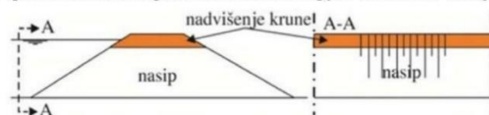
Слика бр. 1: Шематски приказ надвишења круне насипа по целој ширини
