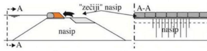
Слика бр. 7: Шематски приказ извођења “зечијег” насипа на круни материјала са лица места
