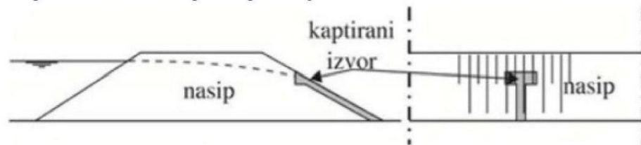
Слика бр. 13: Каптажа извора на брањеној косини насипа
