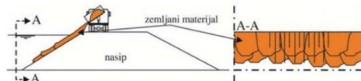
Слика бр. 10: Израда екрана киповањем земљаног материјала
