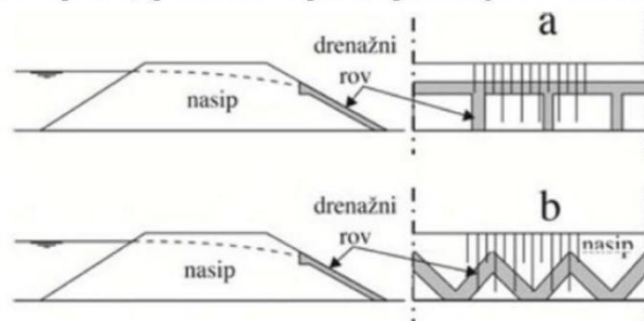
Слика бр. 12: Дренажа извора на брањеној косини насипа
