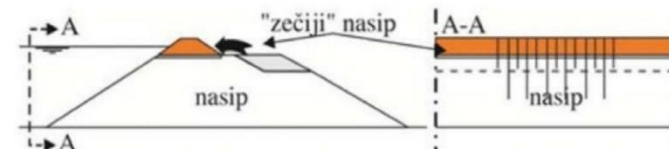
Слика бр. 7: Шематски приказ извођења “зечијег” насипа на круни материјала са лица места
