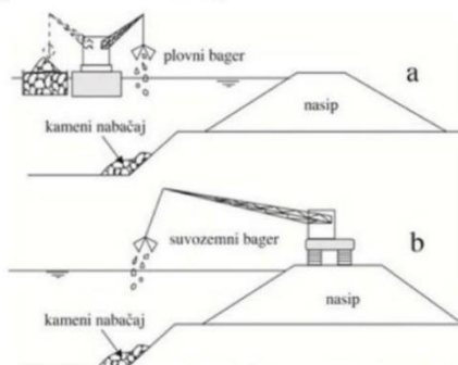
Слика бр.9: Израда каменог набачаја за заштиту обале од ерозије, пловном или сувоземном механизацијом
