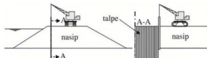
Слика бр. 11: Противфилтрациона завеса од челичних талпи
